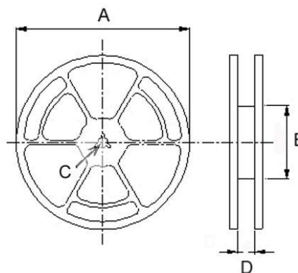
Reel Dimensions
