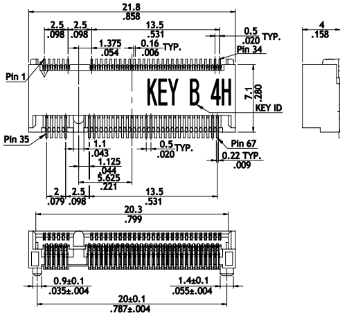
P/N: CS76672AM0-R0
