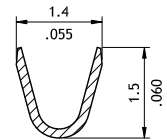
SEC.: A-A
