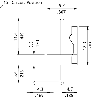
P/N: CI82**P*H00
