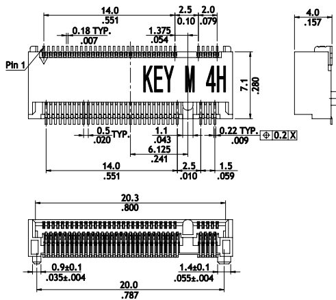
P/N: CS76672AM0-R0
