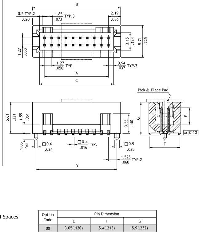
P/N: CHC2***M1**-2*
